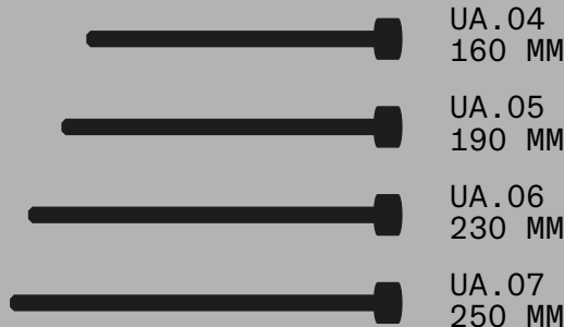
UA.04-07 M10 BOLT
